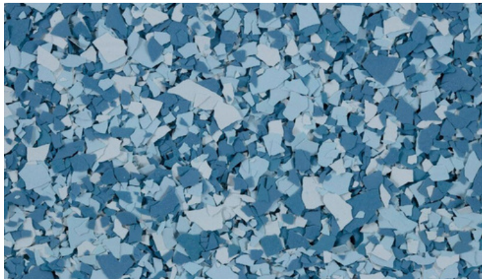
PLUTO
