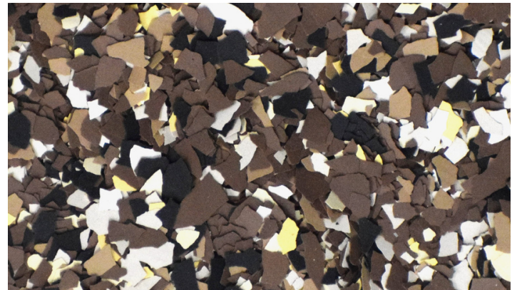
EARTH
